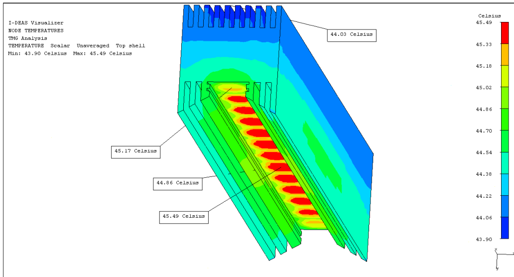
Температура поверхности радиатора
